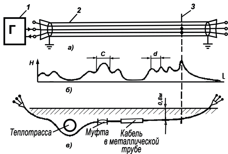
Рис.5.11 КЗ-междуфазное
